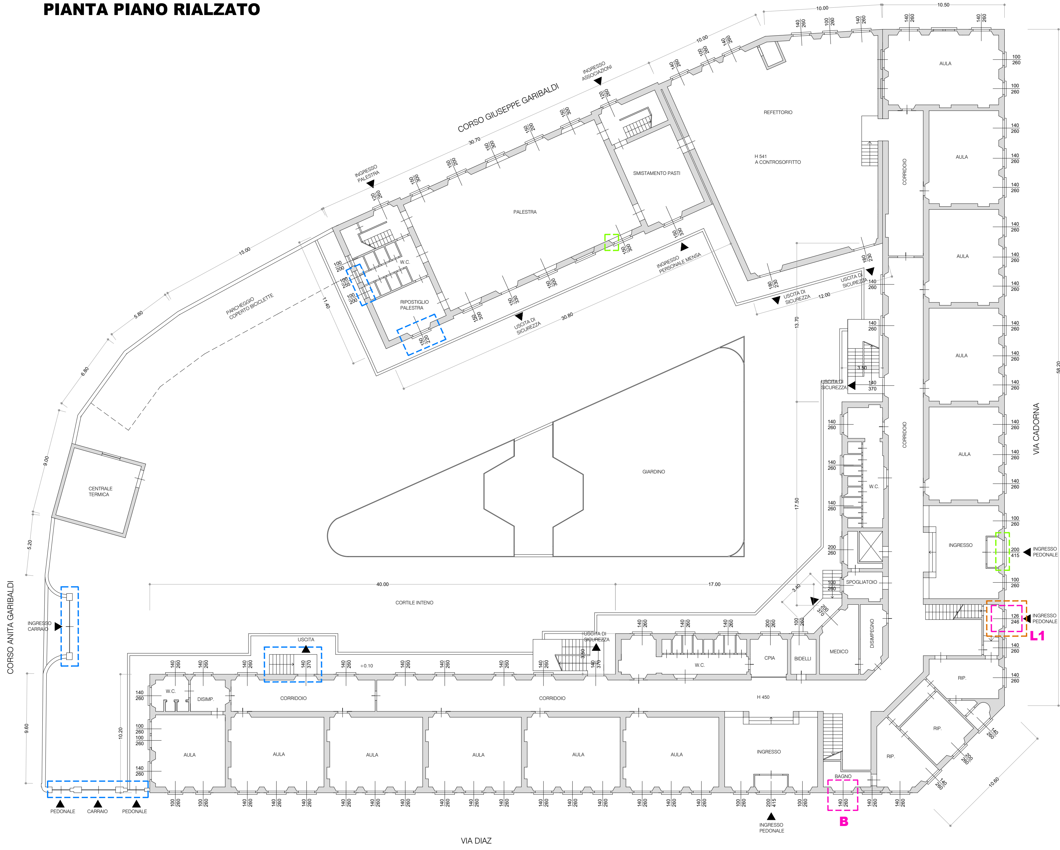
PIANTA PIANO RIALZATO
