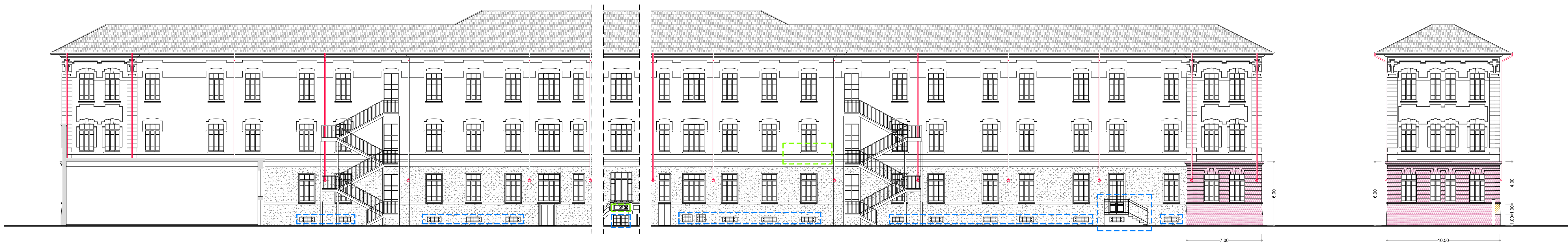
PROSPETTO 4 CORTILE INTERNO
