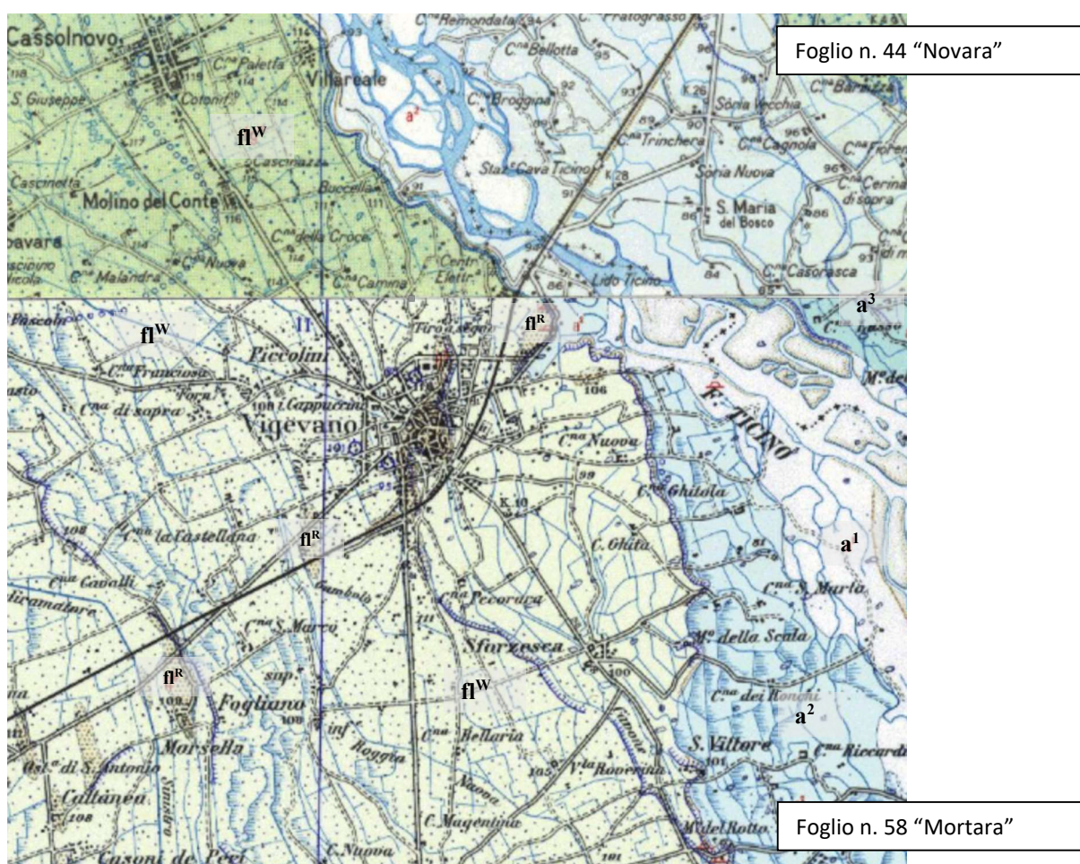
Fig.4.1 – Stralcio Carta Geologica d'Italia – F.44 "Novara" e F.58 "Mortara".
